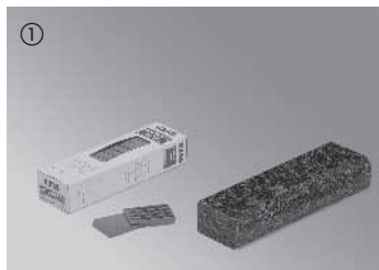
Инструмент для укладки: Брусок, распорные клинья, карандаш, пила.
