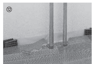
Für aus dem Boden herausragende Heizungsrohre werden in die Elemente Öffnungen (Größe abhängig vom jeweiligen Heizungsrohr und unter Berücksichtigung des erforderlichen Dehnungsabstands) gebohrt und gesägt.
